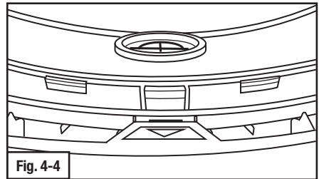
Fig. 4 – Installation du protège-filtre, du pare-étincelles et du préfiltre
