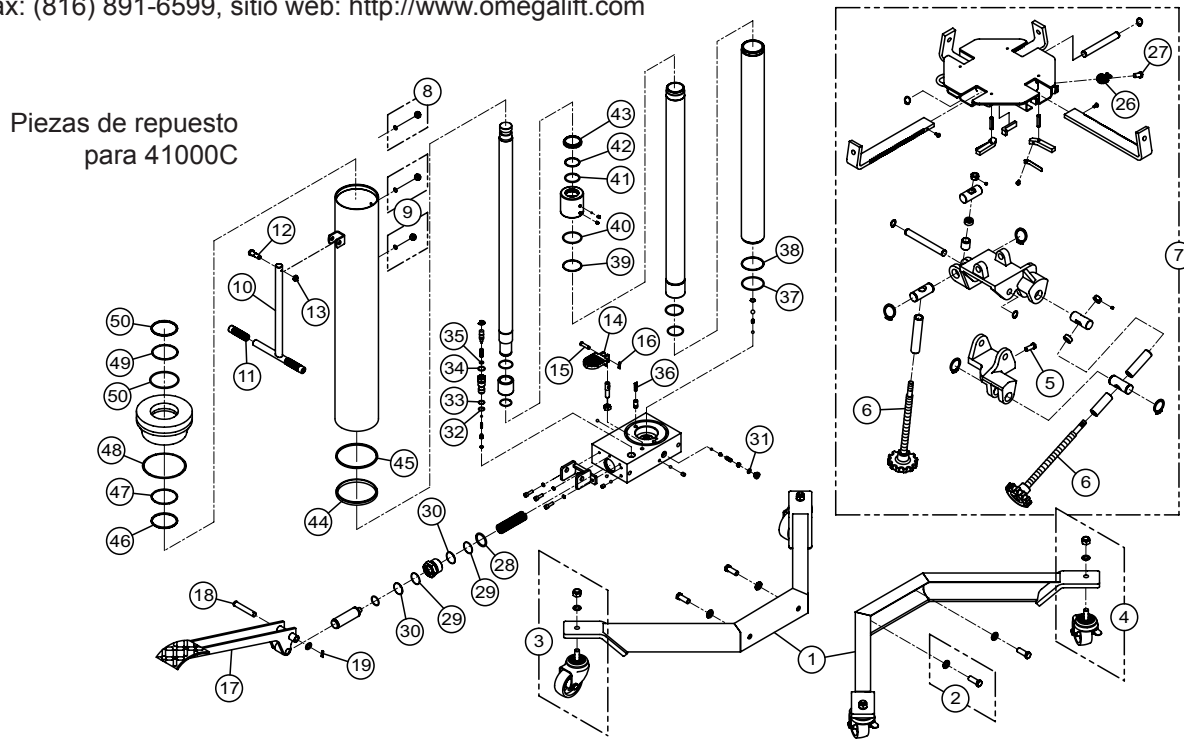
Piezas de repuesto para 41001C
